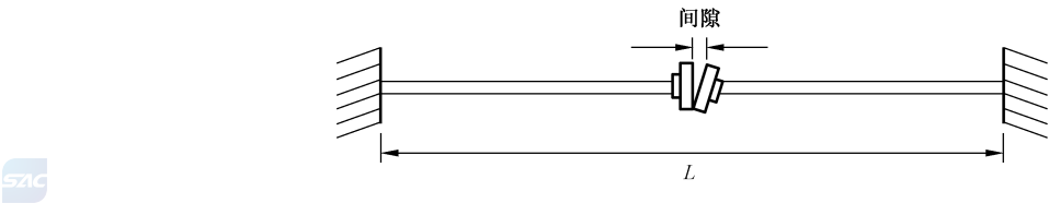
图 A.2 法兰接头组对时的允许间隙
