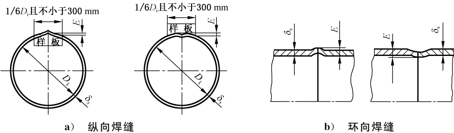
图 2 纵向与环向焊缝处的棱角度检查
